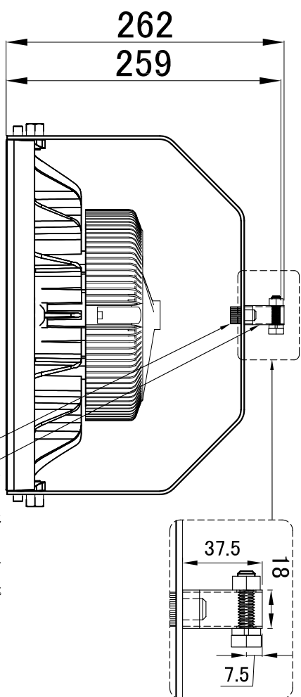
インテリジェントホルダー取付要領図
