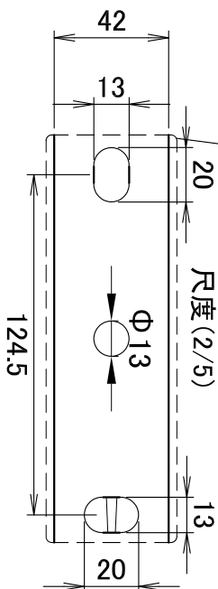
金具取付穴部拡大図
